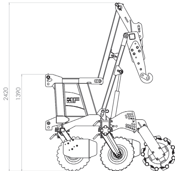
Рис. 6. Вид культиватора сбоку с поднятым гидropaком
