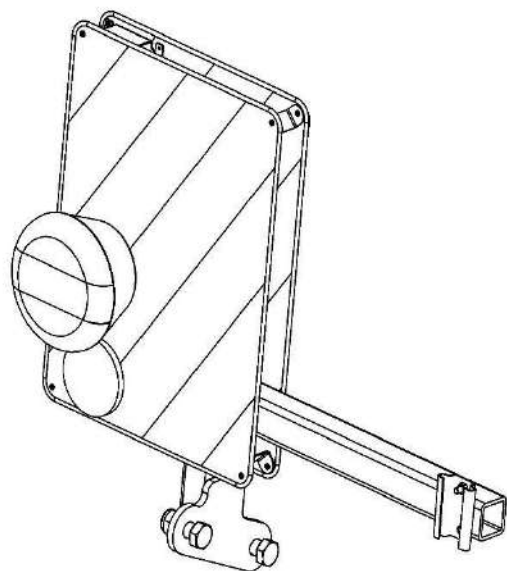
Крепление освещения I (левое) U-740 21.01.00.1
