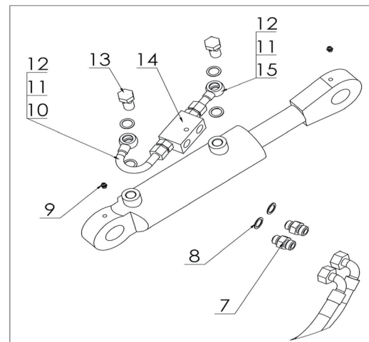
ГИДРАВЛИЧЕСКАЯ СИСТЕМА
