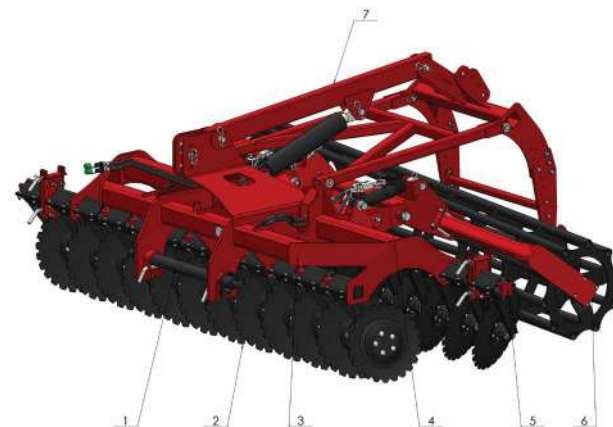
Рис. 3. Конструкция пахотно-посевного культиватора KRUK
