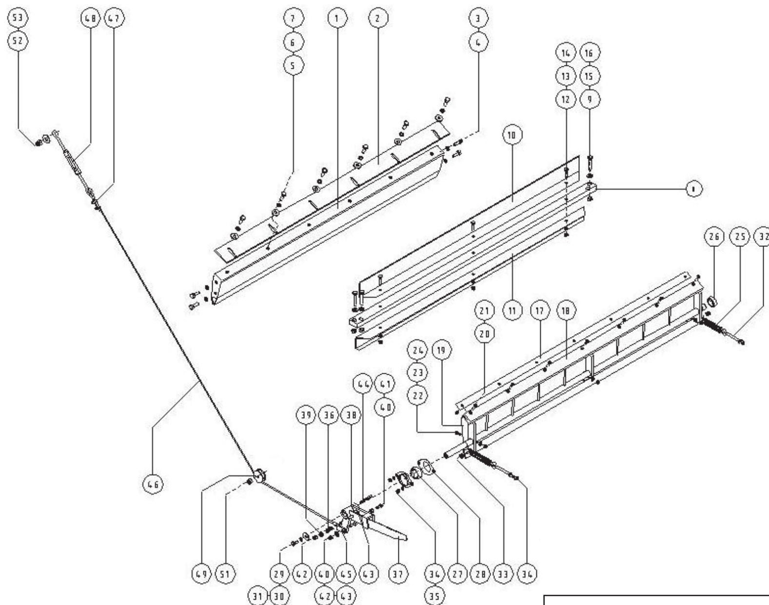
Механизм обвязывания сеткой
