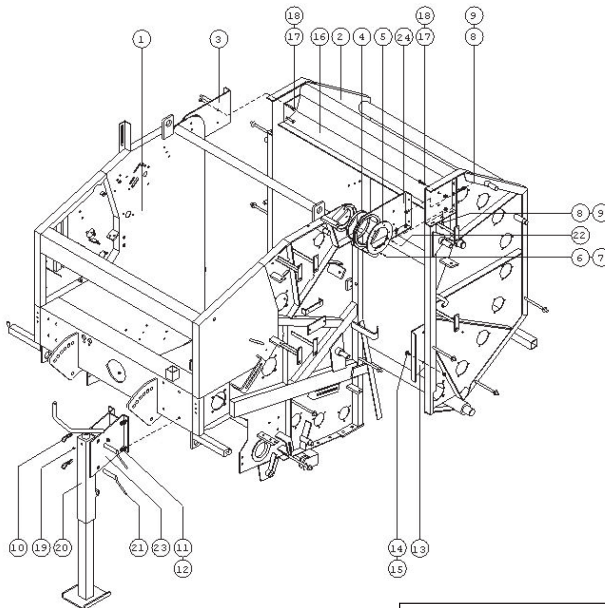
Корпус пресс-подборщика в сборе
