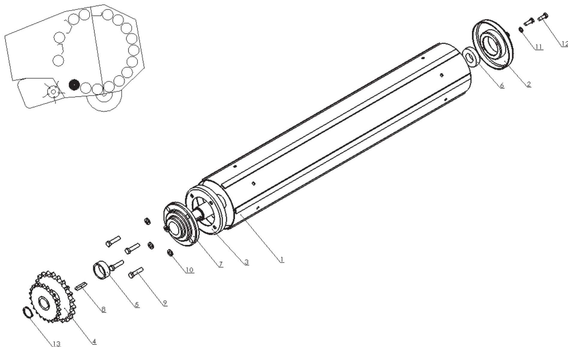
Прессующий вал в сборе VI
