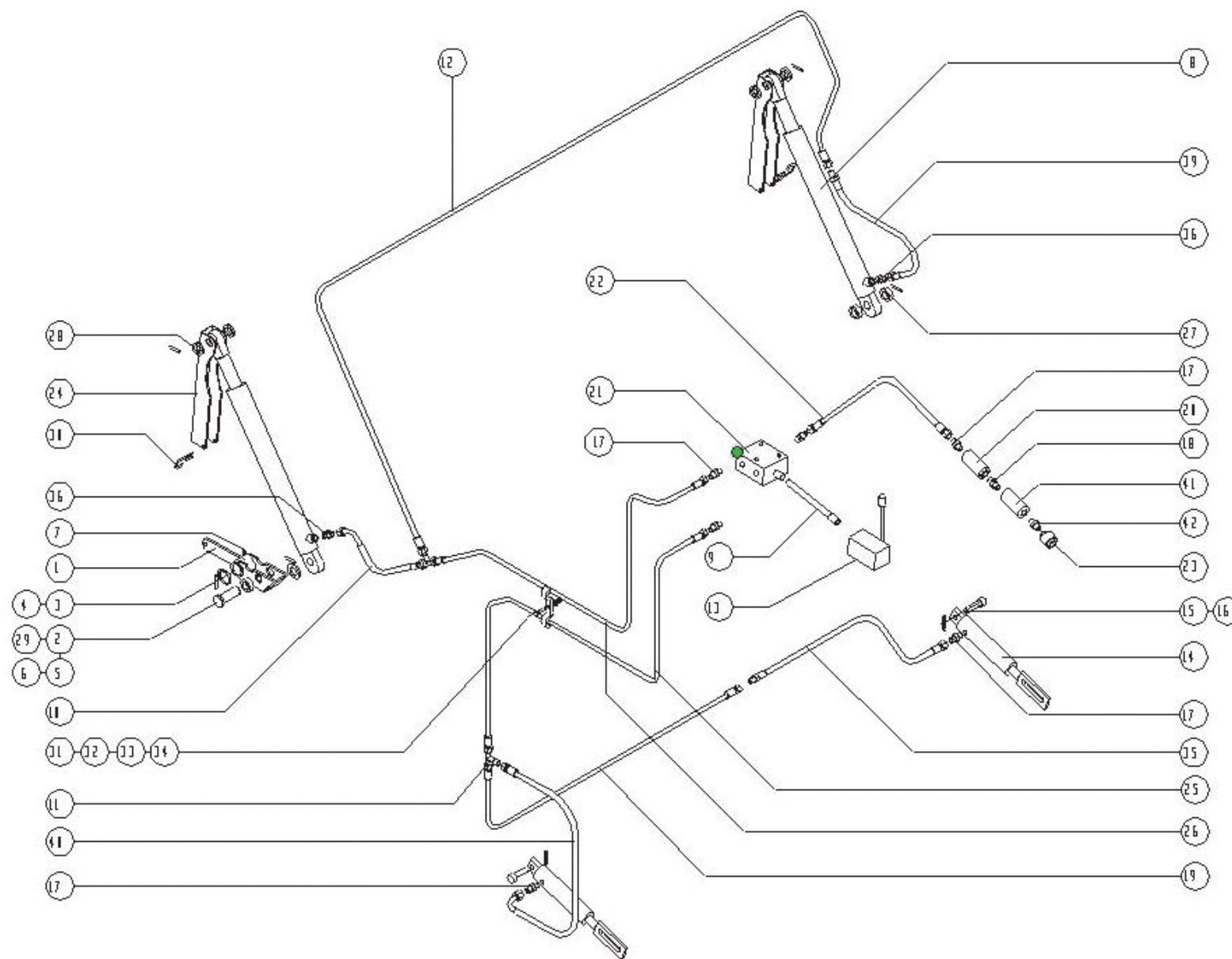
Гидравлическая система
