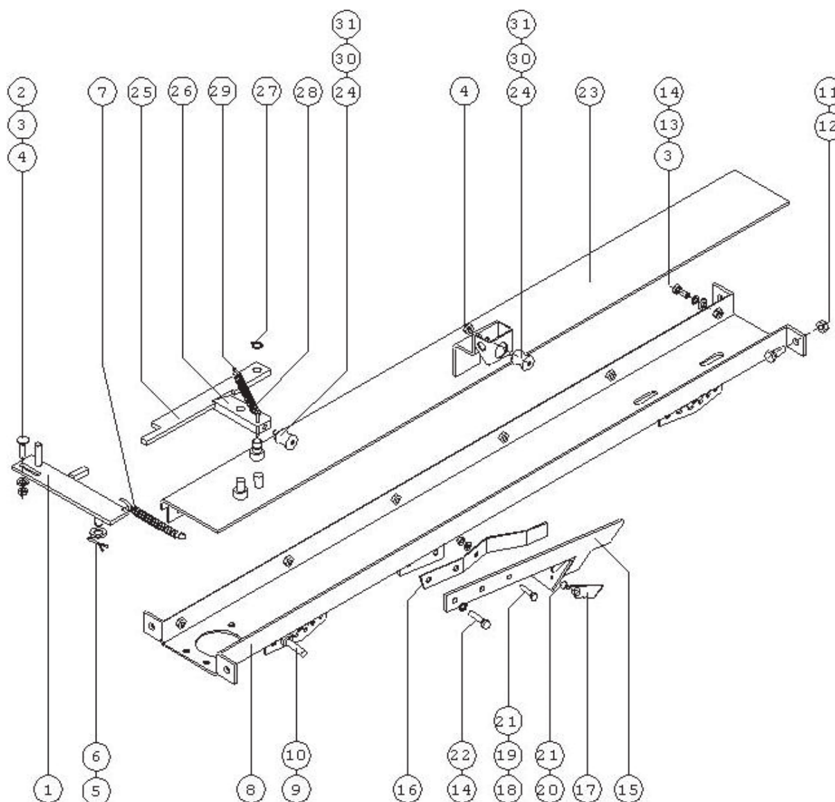
Корпус механизма обвязывания шпагатом
