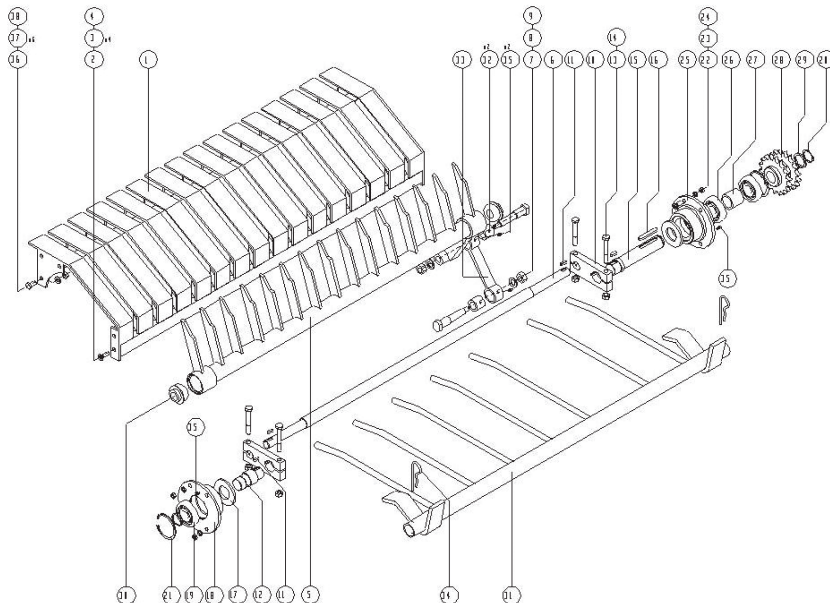
Подборщик в сборе
