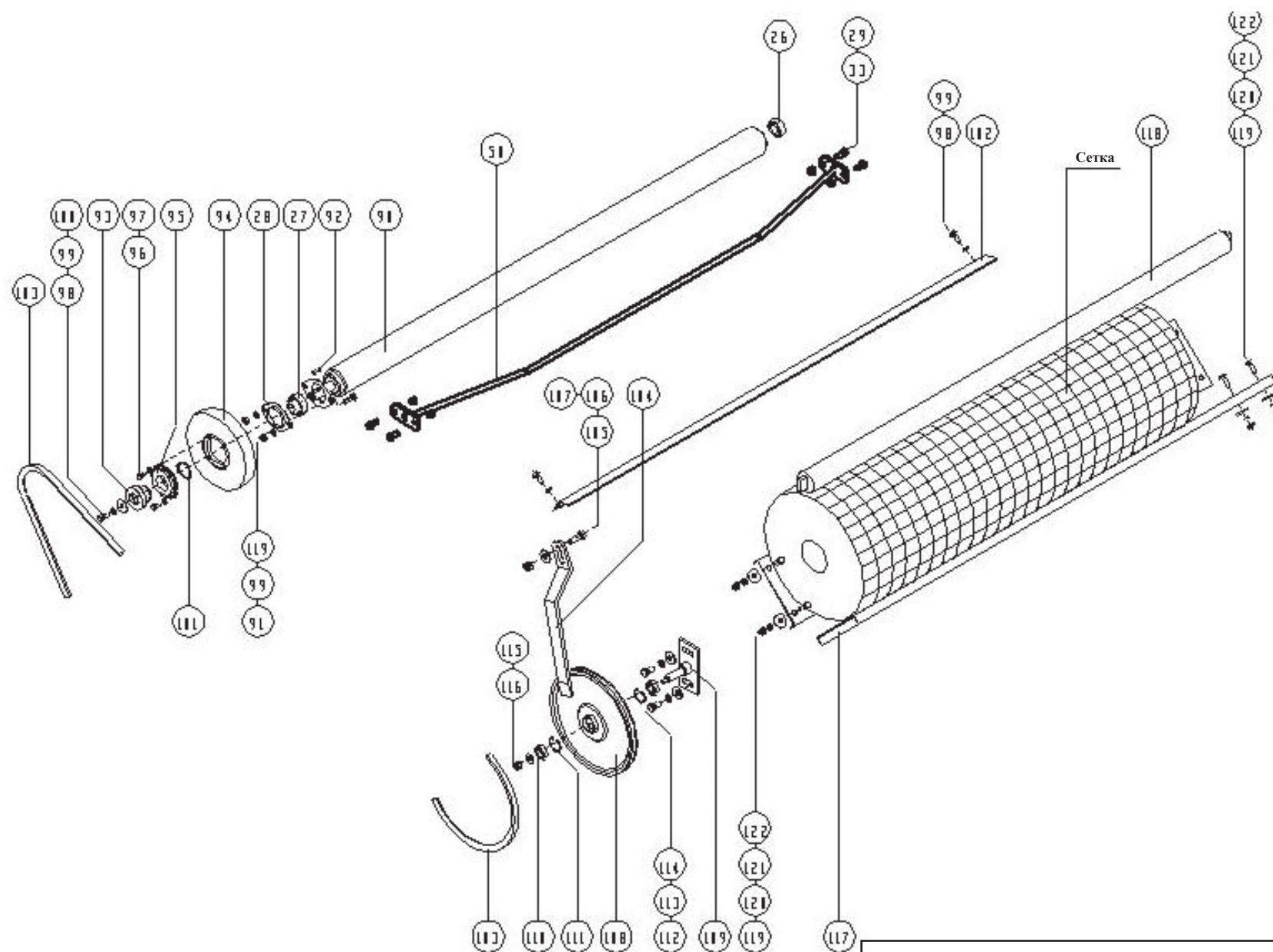
Механизм обвязывания сеткой
