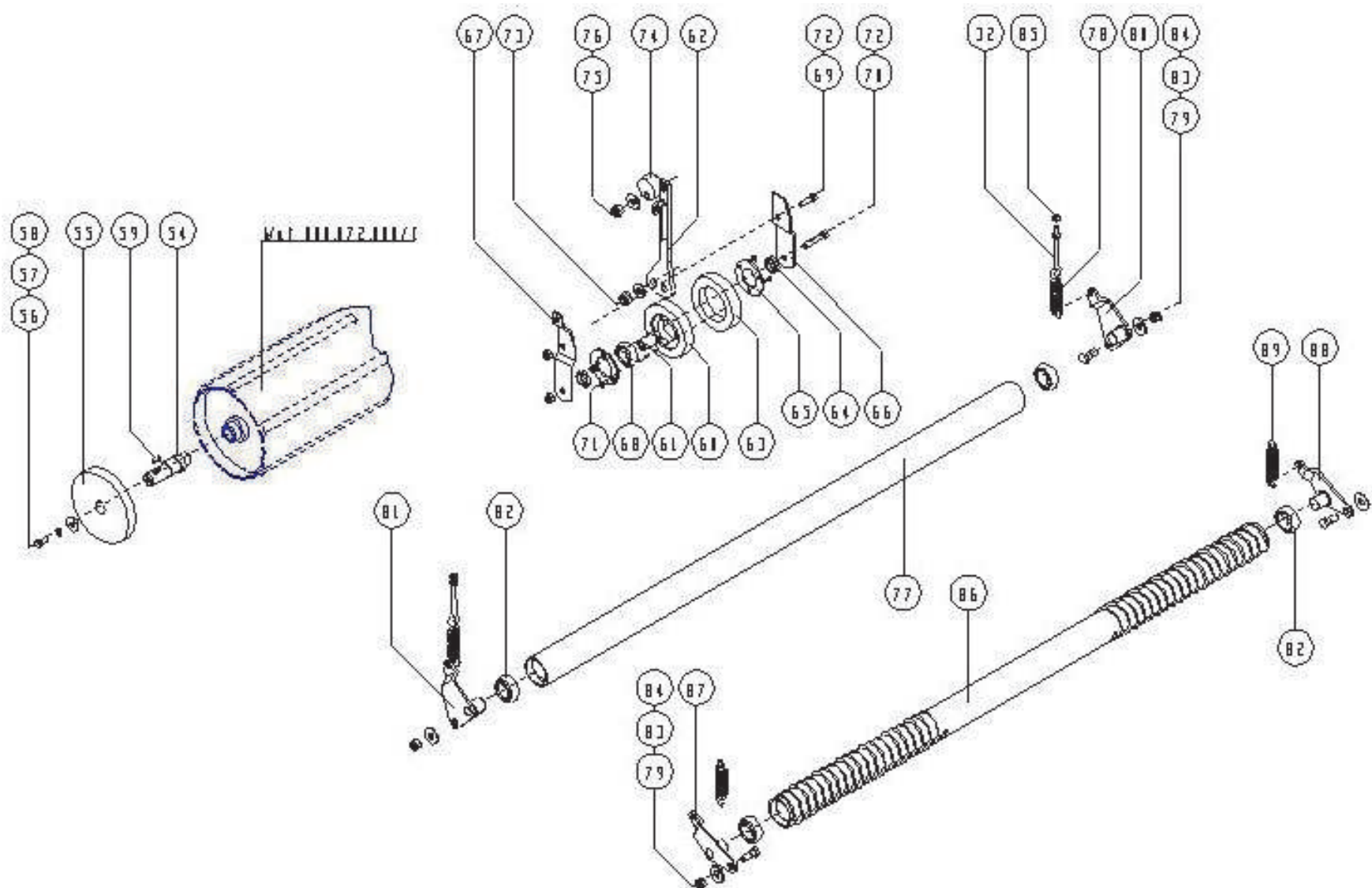
Механизм обвязывания сеткой
