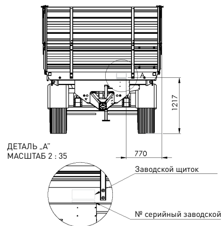
Рис. 2. Место крепления заводского щитка на машине
