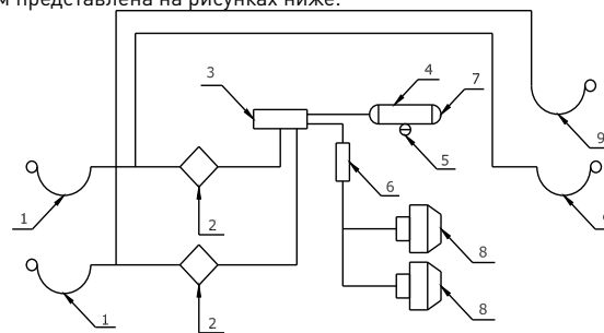
Рис. 5. Схема двухпроводной пневматической тормозной системы. 1 – пневматический соединительный элемент первого прицепа, 2 – воздушный фильтр, 3 – управляющий клапан, 4 – воздушный бак, 5 – водоотводящий клапан, 6 – ручной регулятор силы торможения, 7 – контрольное соединение, 8 – мембранный пневмоцилиндр, 9 – пневматический разъем второго прицепа.
