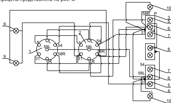
Рис. 4 Схема электрической системы прицепа
