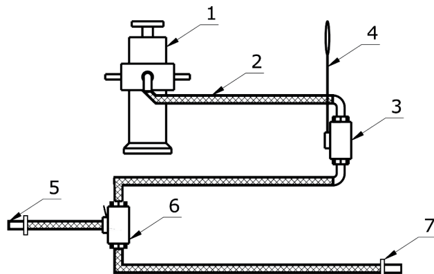
Рис. 3 Схема гидравлической системы механизма опрокидывания грузового кузова
