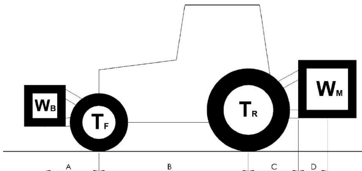
Рис.7. Минимальная нагрузка на переднюю ось трактора
