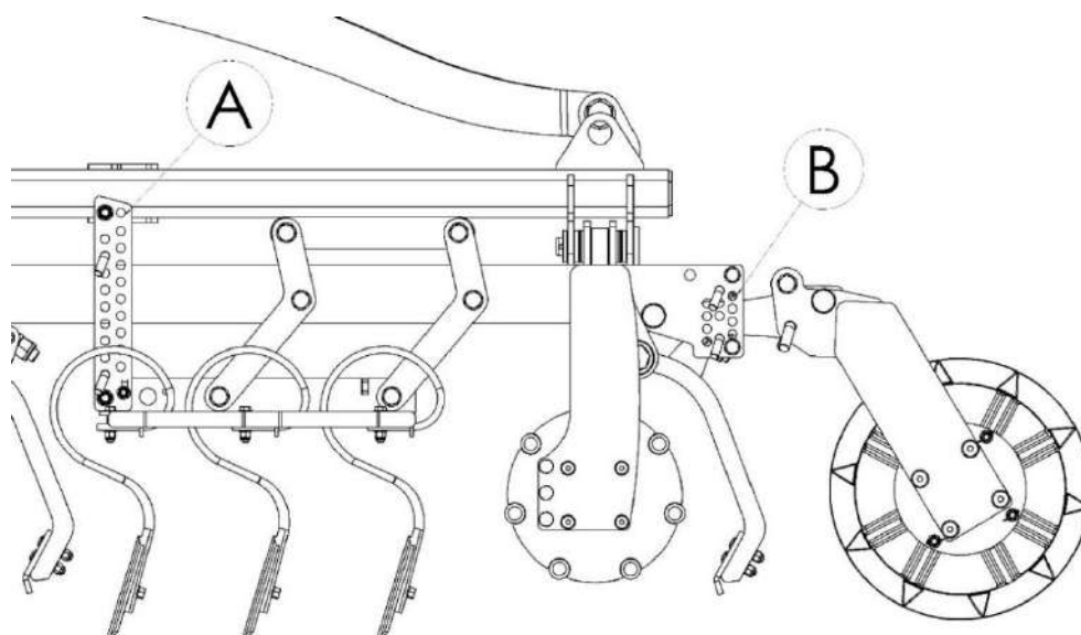
Рис.4. Регулировка рабочей глубины культиватора
