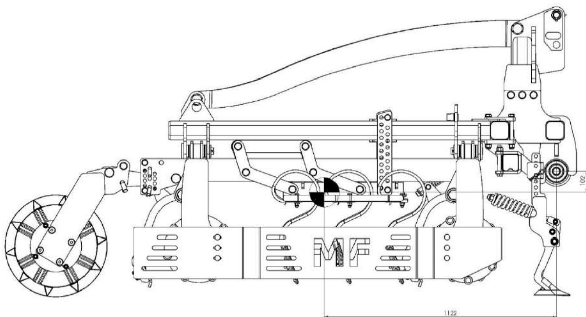
Рис.6. Центр тяжести машины
