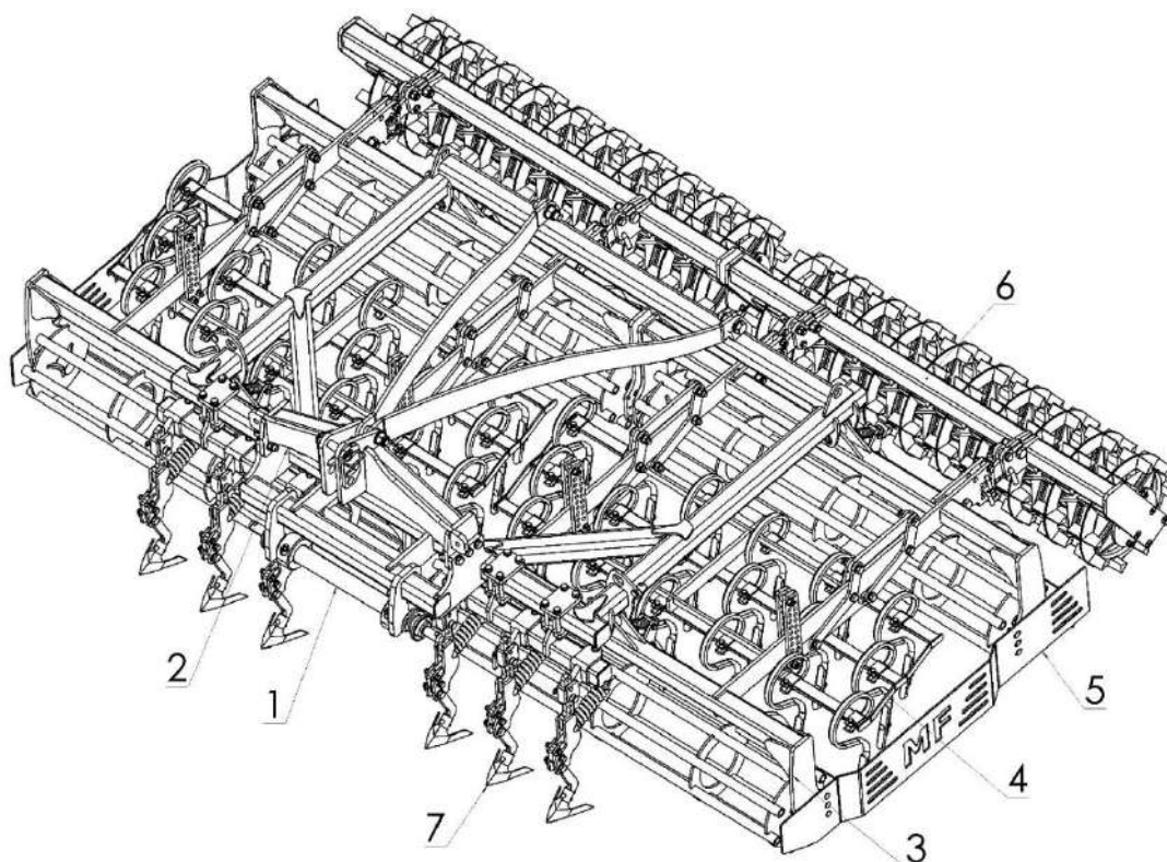
Рис.3. Пружинный предпосевной культиватор балка нижних тяг, 2- рама культиватора, 3- нижняя рама с трубчатыми валами и волокушей, 4- поля рабочих элементов, 5- крайние экраны, 6- прижимающий вал crosskill, 7- следорыхлители (ОПЦИОНАЛЬНО)
