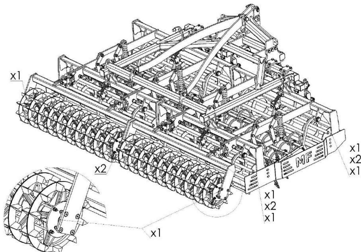
Рис.5. Подшипниковые узлы валов – 12 точек смазки
