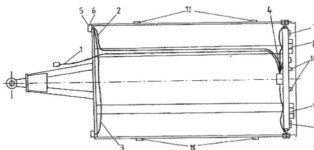
Рис. 3 Схема размещения осветительных приборов прицепа
