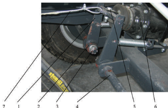
Рис.6. Элементы тормозной системы
