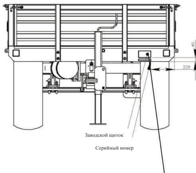
Заводской щиток
