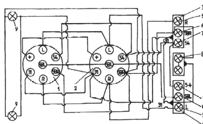
Рис. 2 Схема электрической системы прицепа
