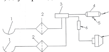
Рис. 4 Схема пневматической тормозной системы
