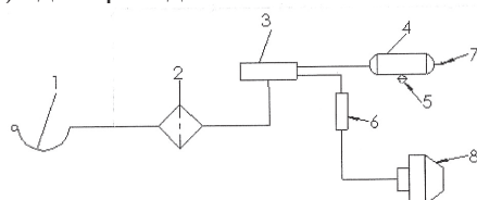
Рис. 4 Схема пневматической тормозной системы
