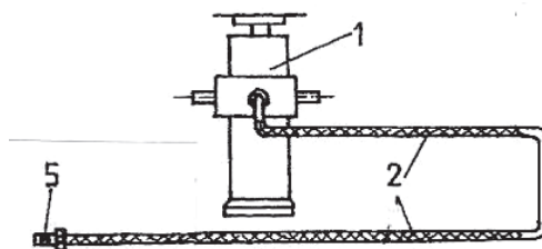
Рис. 1 Схема гидравлической системы механизма опрокидывания грузового кузова
