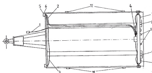
Рис. 3 Схема размещения осветительных приборов прицепа
