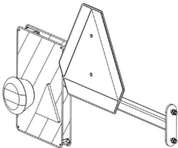
Крепление освещения I (левое) U-710 21.01.00.1
