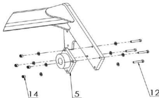
ДЕТАЛЬ «Б»
