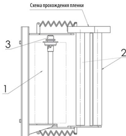
Схема прохождения пленки
