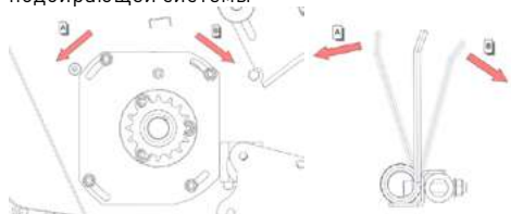
Рис. 34. Регулировка кулачка подборщика.
