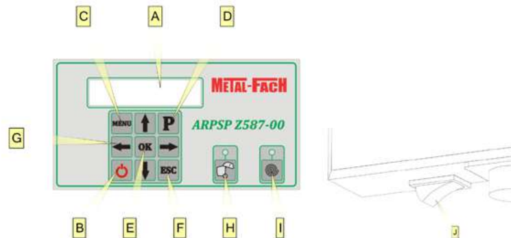
Рис. 17. Панель управления.
