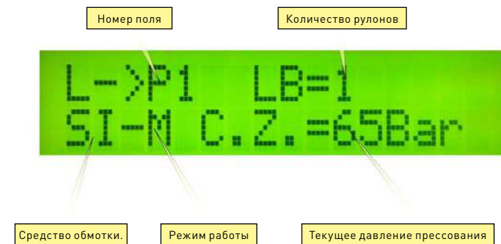
Рис. 18. Главный экран панели управления.
