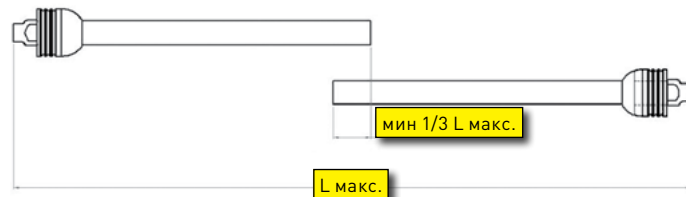
Рис. 9 Длина кожухов BOM
