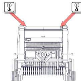
Рис. 48. Точки крепления подвесного устройства.
