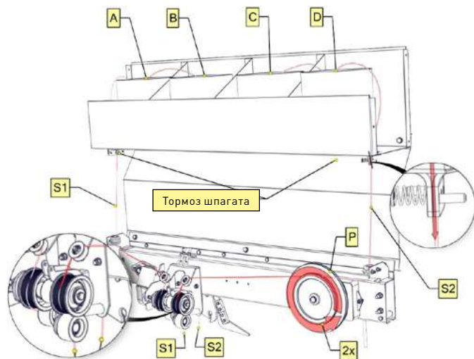
Рис. 14. Установка шпагата
