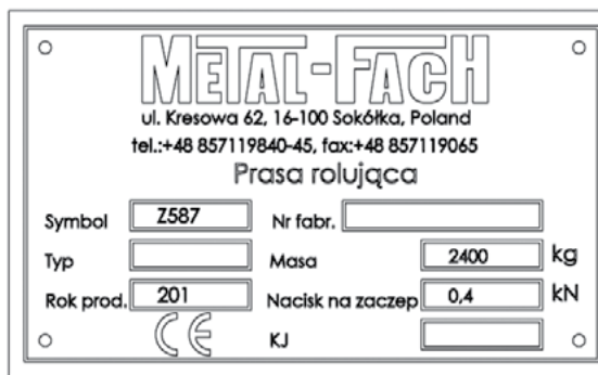
Рис. 1. Заводской щиток
