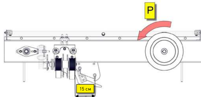
Рис. 13. Элемент, направляющий шпагат
