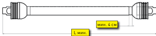
Рис. 8 Длина BOM
