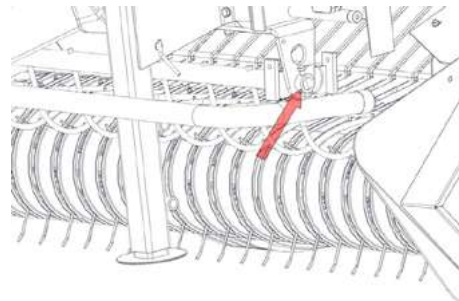
Рис. 21. Демонтаж прижима укоса
