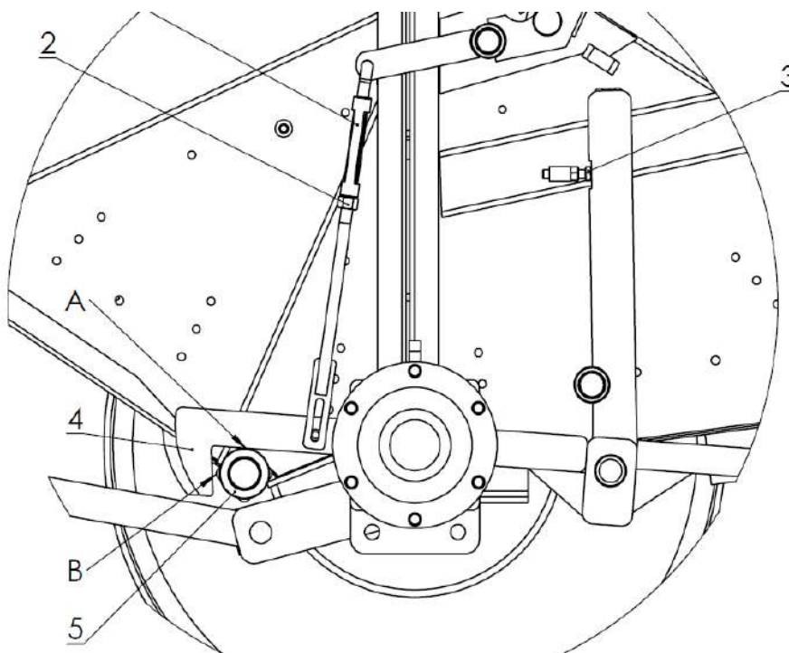
Рисунок 19. Регулировка замка
