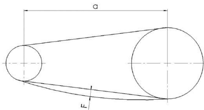
Рисунок 5. Натяжение цепи
