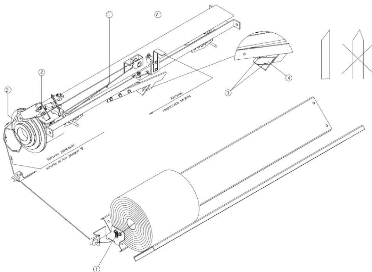
Рисунок 15. Путь шпагата
