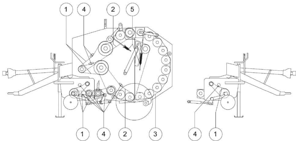
Рисунок 6. Приводной узел
