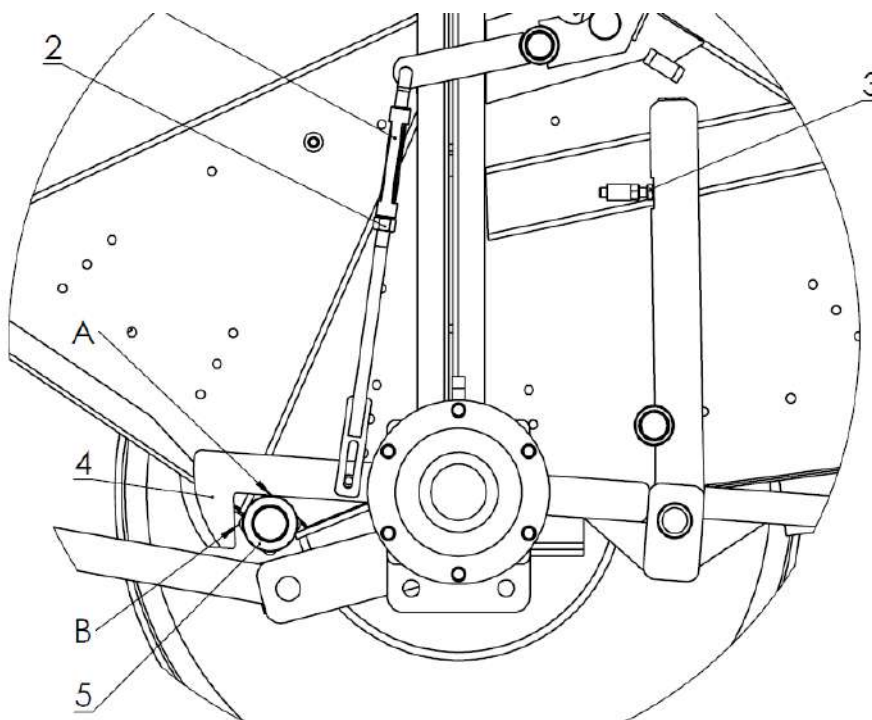
Рисунок 19. Регулировка замка
